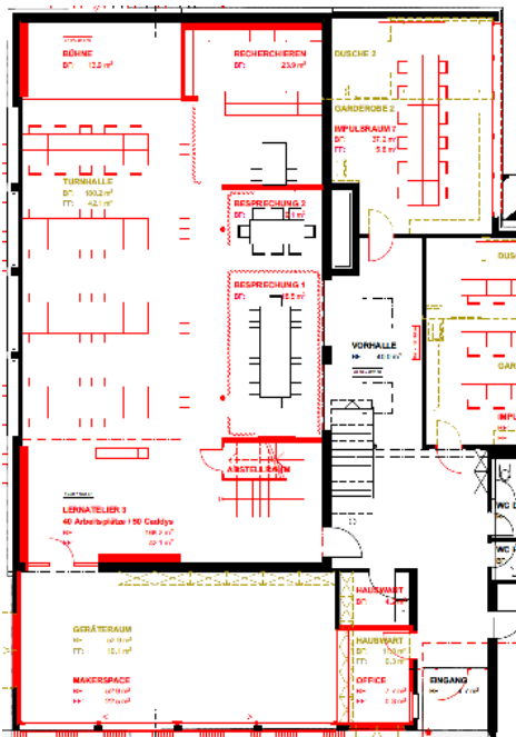
Bauplan: Erdgeschoss Turnhallentrakt
